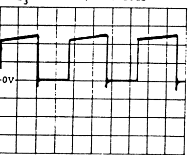
555 Pin 7 5V/DIV. 10uS
