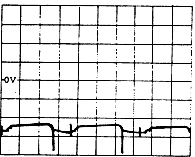
Q 3 Base 10V/DIV. 10uS
